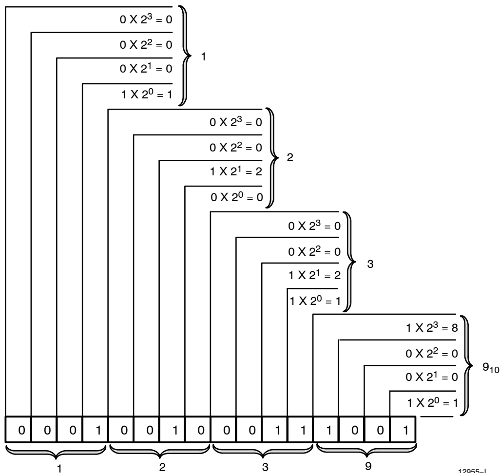
図C.1 4桁のBCD
