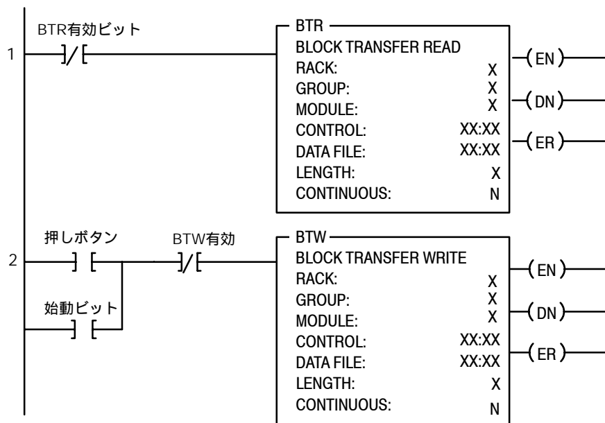
図3.3 PLC-5ファミリーのプログラム例の構造
